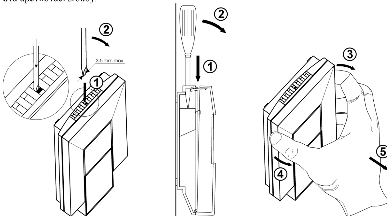
Obrázek 2: Demontáž snímače
