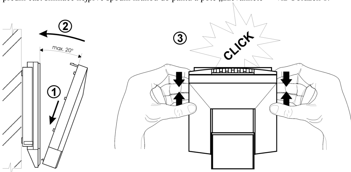
Obrázek 1: Montáž snímače
